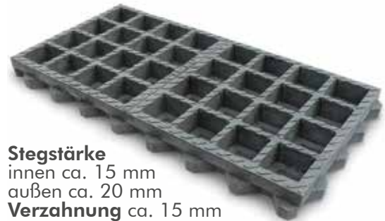
TTE MultiDrain PLUS OBERSEITE
